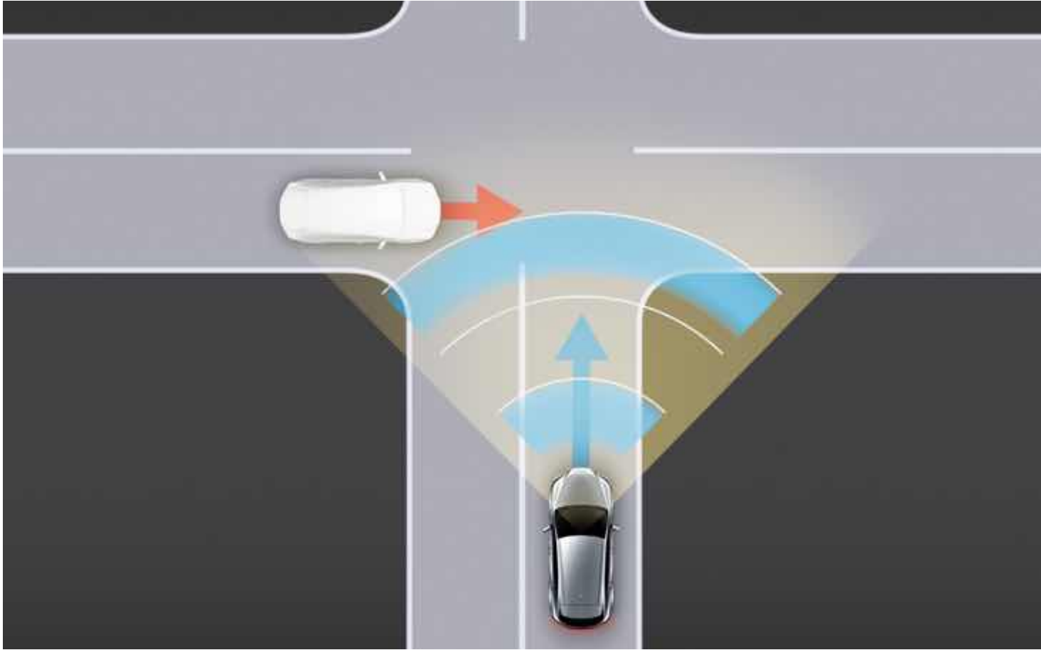
预碰撞安全系统PCS带紧急转向辅助功能ESA
